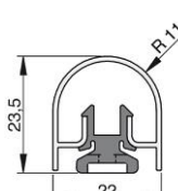
BU-22K
