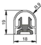
BU-18K
