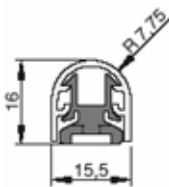
BU-16K
